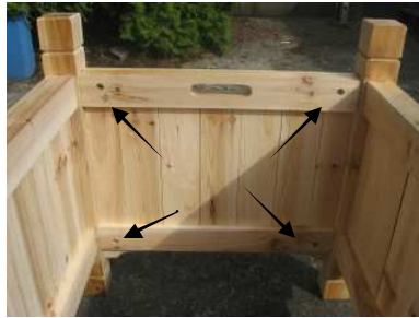
Fig. 1. Insert Nuts
